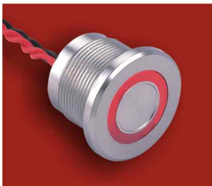
PS223P□Y◆1△▲ Panel size 安装孔尺寸: \Phi 22\text{mm} IP degree 防护等级: IP68, IK10
